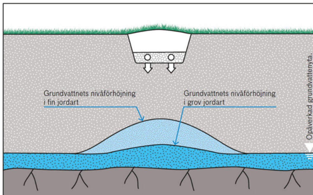
Figur 2. Grundvattennivån kommer att höjas under en infiltration i fin jordart.
