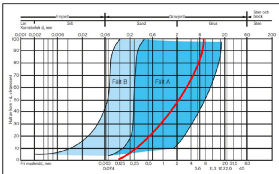
Figur 3. Siktanalys som visar att jordarten på platsen för planerad infiltration ligger i fält A, vilket innebär att tillägg för förhöjning under infiltrationen inte behöver göras. FH_{inf}=0
