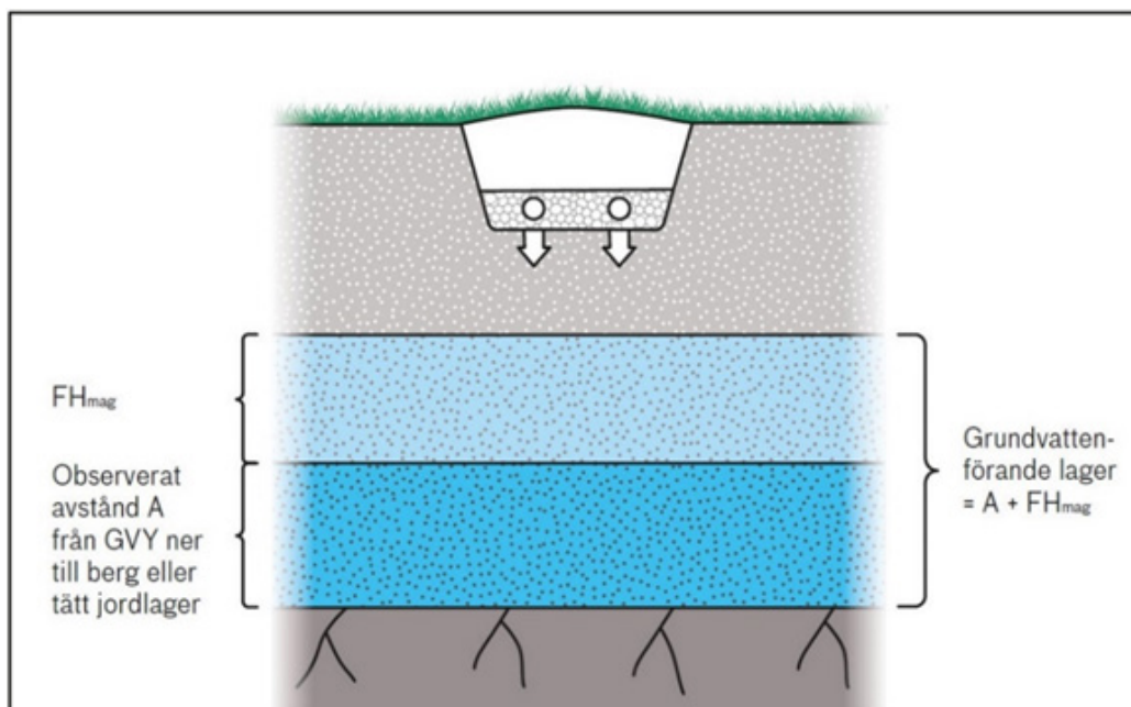
Figur 4. Principskiss över grundvattenförande lager. Har man räknat fram en korrigerad nivå för FH_{mag} så kan beräkningen av grundvattenförande lager beskrivas som denna nivå minus jorddjupet/avstånd till tät jordlager.
