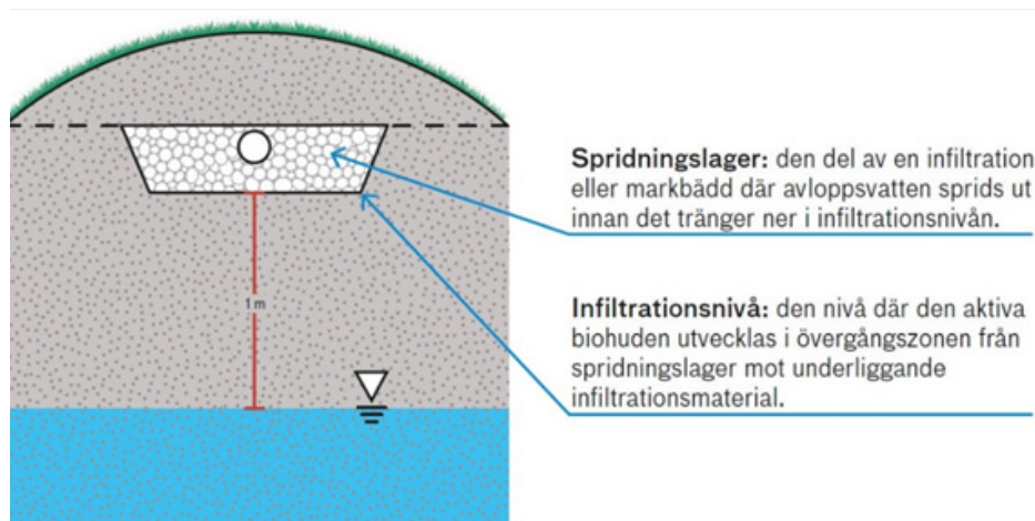
Figur 1. För att reningen i en infiltrationsanläggning ska fungera ska avståndet mellan infiltrationsnivån och den högsta dimensionerande grundvattennivån (den omättade zonen) vara minst 1 meter under större delen av året.
